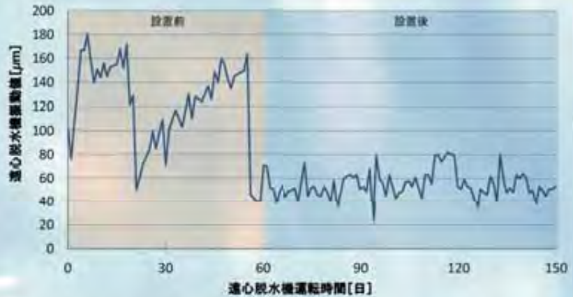
遠心脱水機 振動値の推移
